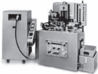
Výsledek první zakázky z 13. května 1962: plně automatický rovnač stroj VRJ IIa
